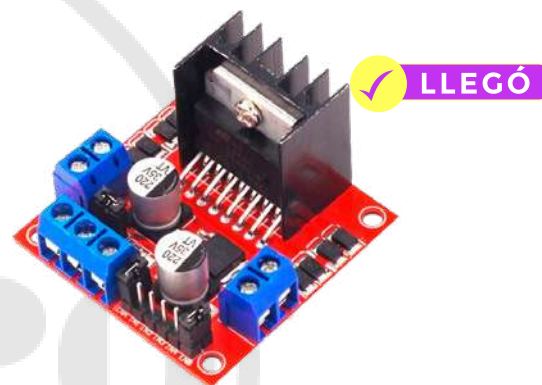
MÓDULO CONTROLADOR MOTOR L298N -DOBLE PUENTE H
