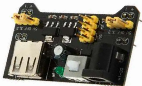
MÓDULO FUENTE DE PODER 5V-3.3V
