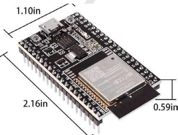
PLACA DE DESARROLLO IOT ESP32 - 38 PINES
