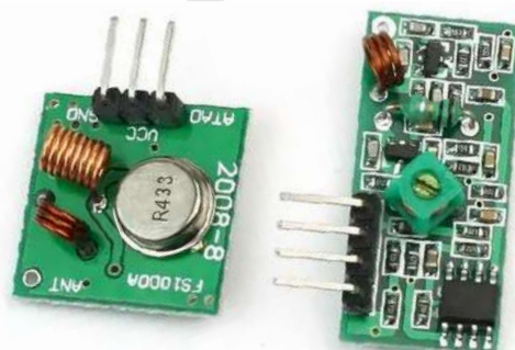
MÓDULO RF433 TRANSMISOR RECEPTOR
