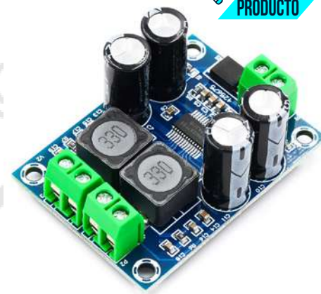
MODULO AMPLIFICADOR DE AUDIO XH-M311
