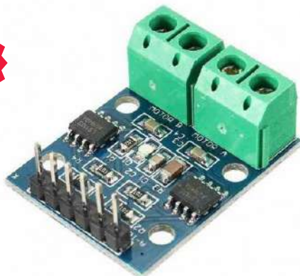
MÓDULO CONTROLADOR PASO A PASO DOBLE
