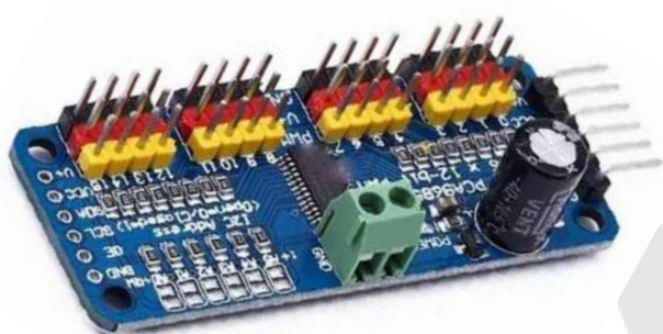
MODULO CONTROLADOR DE MOTOR CON 16 SALIDAS PWM SERVOMOTOR ARDUINO
