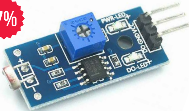
MODULO SENSOR DE LUZ LDR FOTOCELDA
