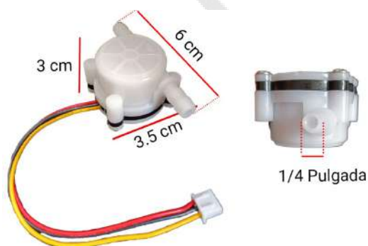
SENSOR CAUDAL DE AGUA -(.3-6L/min) Cod. ARD-SCAUDAL
