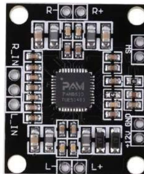
AMPLIFICADOR PAM8610 2X15W ARDUINO
