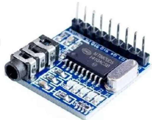
DECODIFICADOR DE VOZ DTFM MT8870
