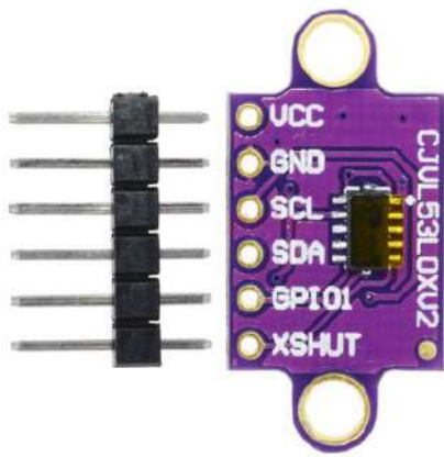
SENSOR DE DISTANCIA LASER VL53L0X GY VL53L0XV2 ARDUINO
