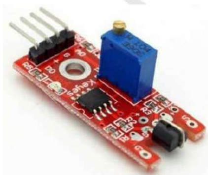
MÓDULO EFECTO HALL
