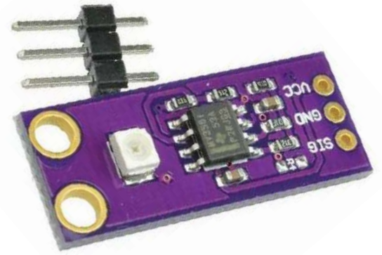
SENSOR INTENSIDAD LUZ ULTRAVIOLETA UV GUA-S12S ARDUINO
