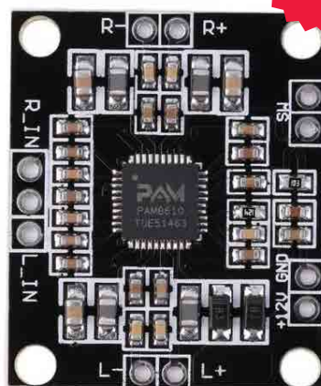
AMPLIFICADOR PAM8610 2X15W ARDUINO
