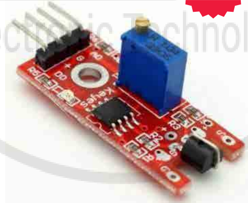
MÓDULO EFECTO HALL SENSOR DE CAMPO MAGNETICO CON GRADUACION KY-024 49E
