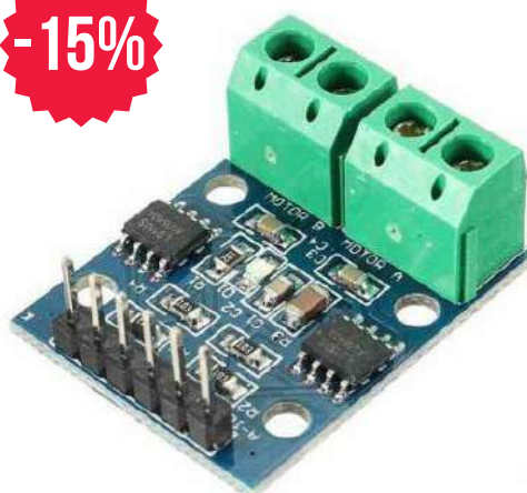
MÓDULO CONTROLADOR PASO A PASO DOBLE
