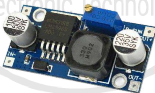
MÓDULO LM2596 CONVERTIDOR
