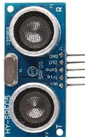
MÓDULO ULTRASONIDO ARDUINO HC-SRF05
