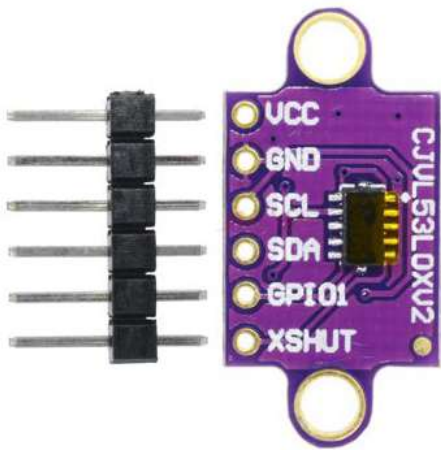
SENSOR DE DISTANCIA LASER VL53L0X GY VL53L0XV2 ARDUINO
