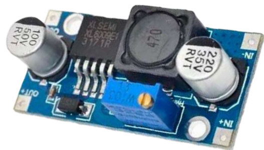
MÓDULO FUENTE ELEVADORA DC 5-32V
