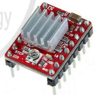
MODULO MOTOR PASO A PASO A4988
