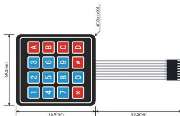
TECLADO 4X4 MATRIZ
