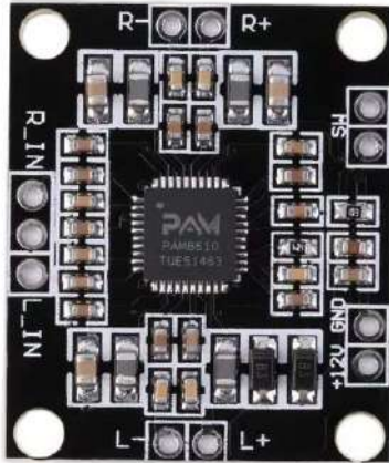
AMPLIFICADOR PAM8610 2X15W ARDUINO
