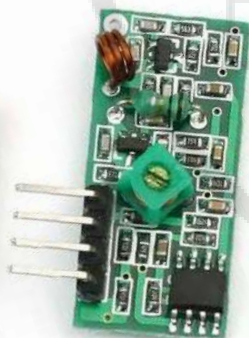
MÓDULO RF433 TRANSMISOR RECEPTOR
