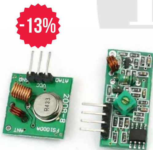
MÓDULO RF433 TRANSMISOR RECEPTOR
