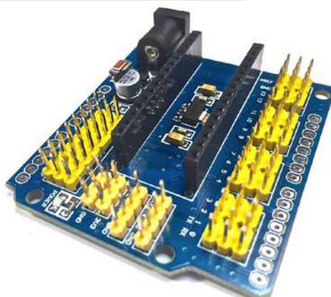
MÓDULO EXPANSIÓN ARDUINO NANO
