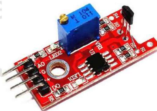
MÓDULO EFECTO HALL SENSOR DE CAMPO MAGNETICO CON GRADUACION KY-024 49E
