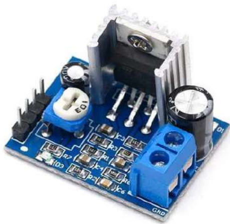
MÓDULO AMPLIFICADOR AUDIO TDA2030A
